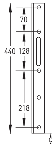
Für Heizkörper Höhe 740 und 990 mm
