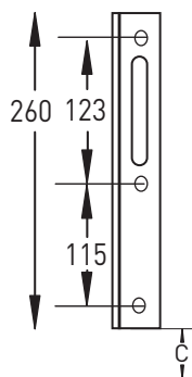
Für Heizkörper Höhe 440, 500 und 590 mm
