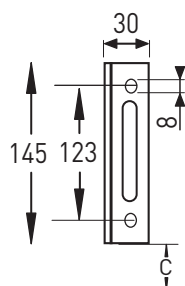
Für Heizkörper Höhe 300 mm
