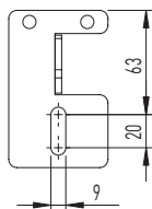
Wandhalterung, Profilsansicht
