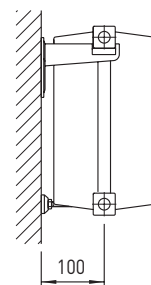
SCD, Typ 24 oder 26 profilansicht
