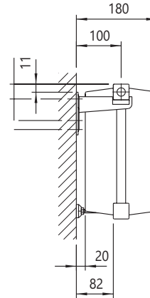
SC doppelagig (SCD), typ 24 oder 26 Profilansicht
