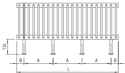
Heizkörper mit 4 Standfüße SF124
