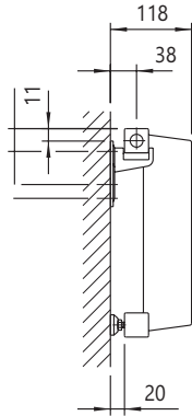
SC einlagig (SCE), typ 14 oder 16 Profilansicht
