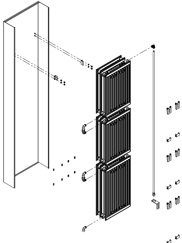
Zeichnung 8.4
