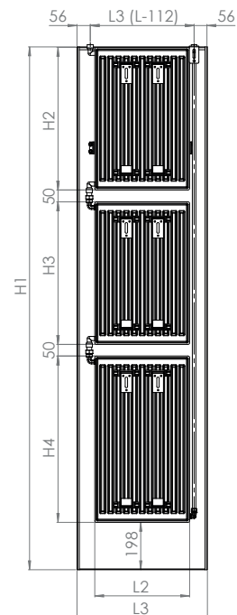
Zeichnung 6.2
